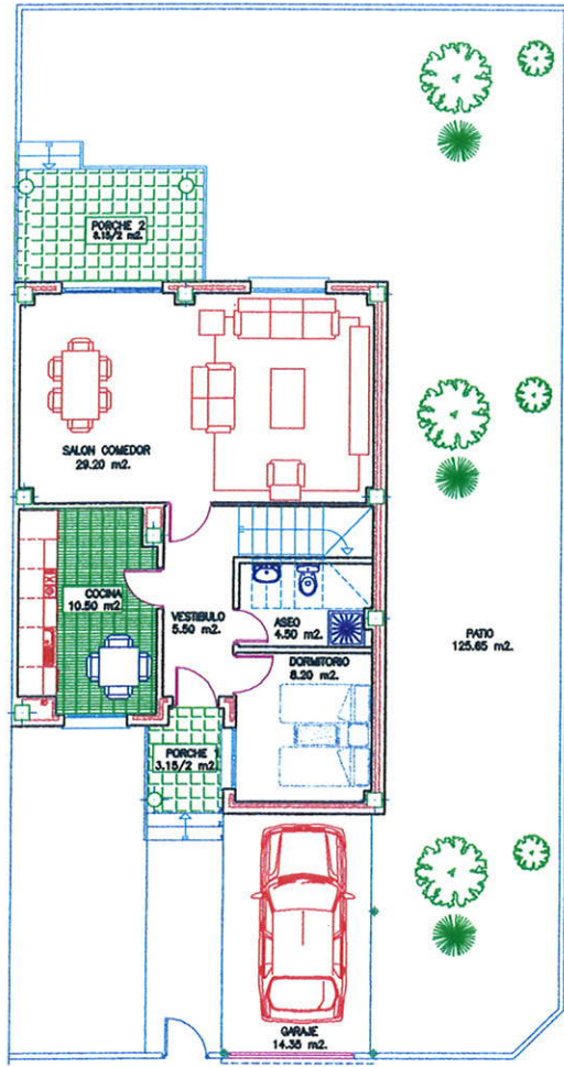
Planta Baja.
