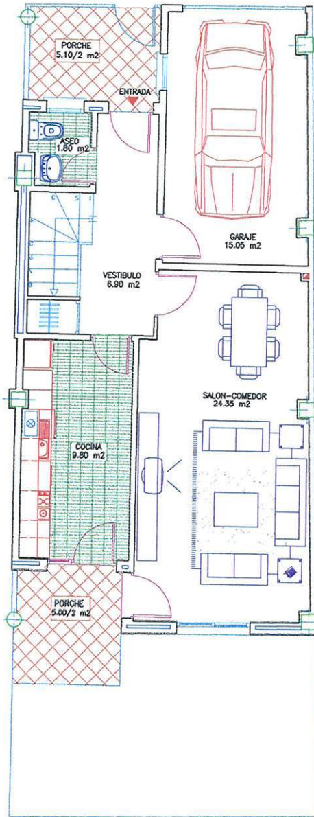
PLANTA BAJA
