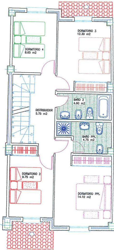
PLANTA PRIMERA
