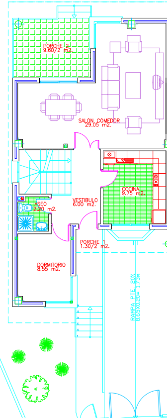
Planta Baja
