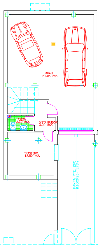
Planta Sotano
