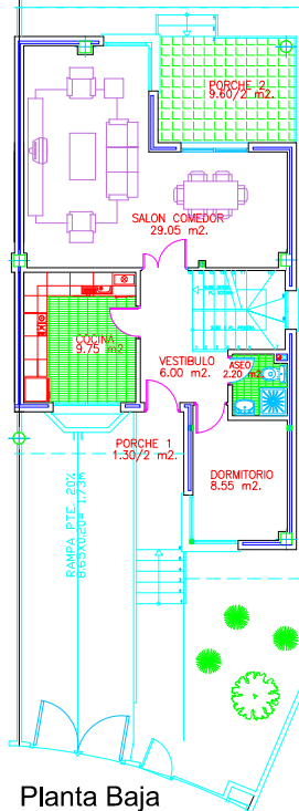
Planta Baja
